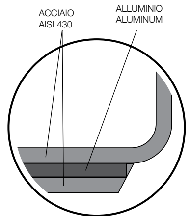
Fondo termodiffusore Thermal diffusion bottom
